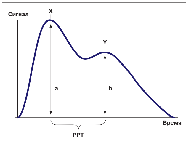
Рис. 1. Схема формирования цифровой пульсовой волны
